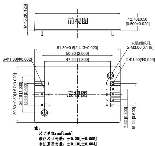
标准封装
