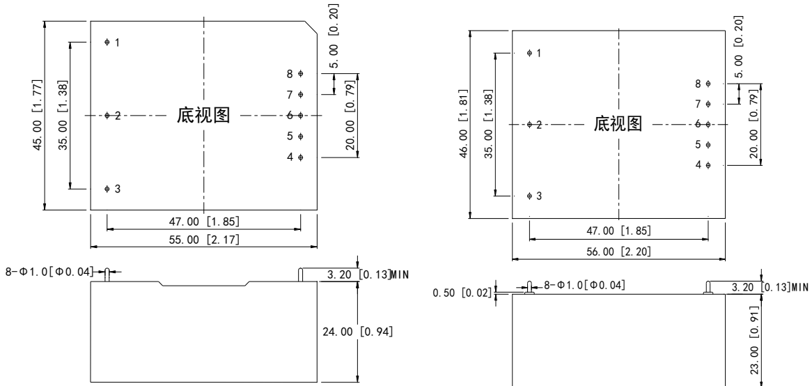
塑料壳尺寸
