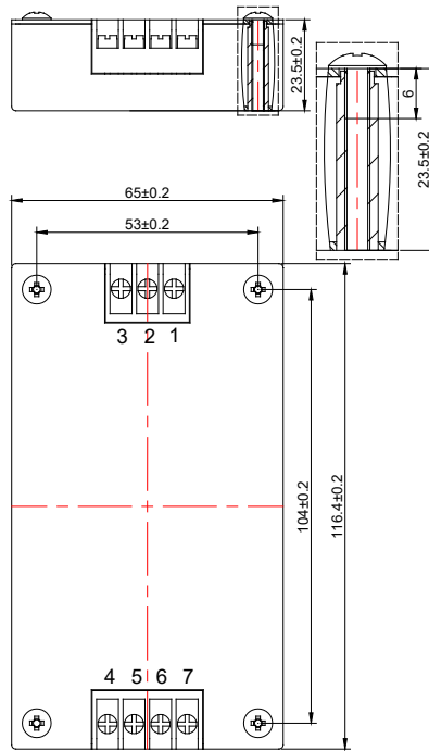
图1 (产品尾缀不带DB) 产品尺寸 (长宽高) 为 116.4*65*23.5mm
