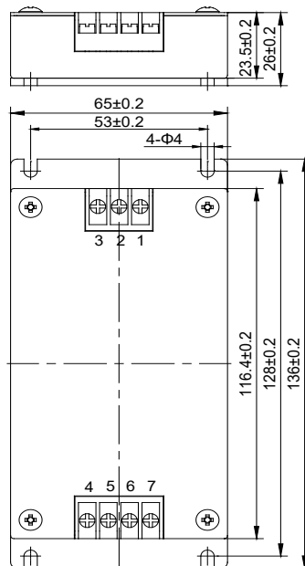
图2 (产品尾缀带DB) 产品尺寸 (长宽高) 为 136*65*26mm
