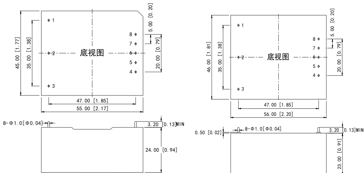
塑料壳尺寸
